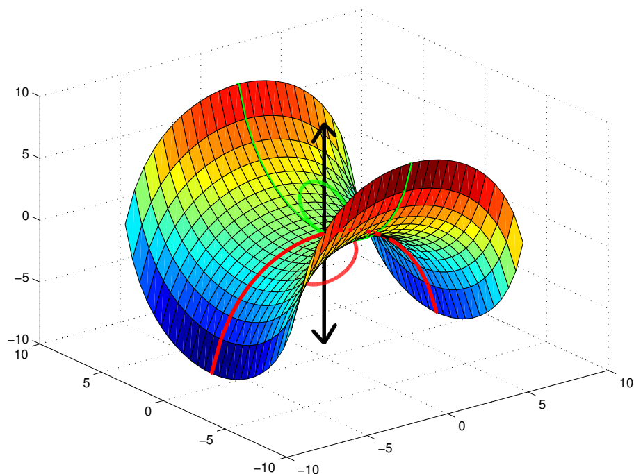
Abbildung 2: Zwei Kurven maximaler Krümmung auf der Scherk'schen Minimalfläche, mit Krümmungskreisen und antagonistischen "Kräften"
