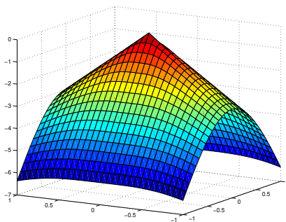
Abbildung 8: Die Funktion -\frac{\partial^2 u}{\partial^2 x} mit Singularität im Nullpunkt
