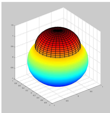
Abbildung 6: Einschränkung auf das unsichtbare Kugelsegment, das innerhalb der aufgesetzten Halbkugel liegt
