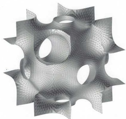
Abbildung 5: Eine etwas exotischere Fläche konstanter mittlerer Krümmung, dreifach periodisch, hier nur der Fundamentalbereich im Einheitswürfel
