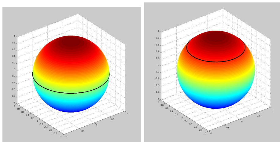
Abbildung 4: Flächen konstanter mittlerer Krümmung: Zwei Halbkugeln oder zwei Kugelsegmente, die jeweils von einem Kreis berandet sind
