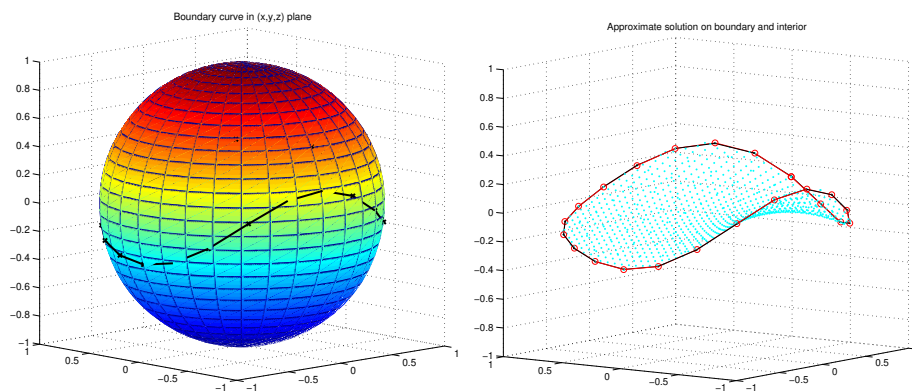
Abbildung 7: Eine Fläche mit H = 0.2 innerhalb der Einheitskugel zu gegebener Randkurve auf der Einheitskugel
