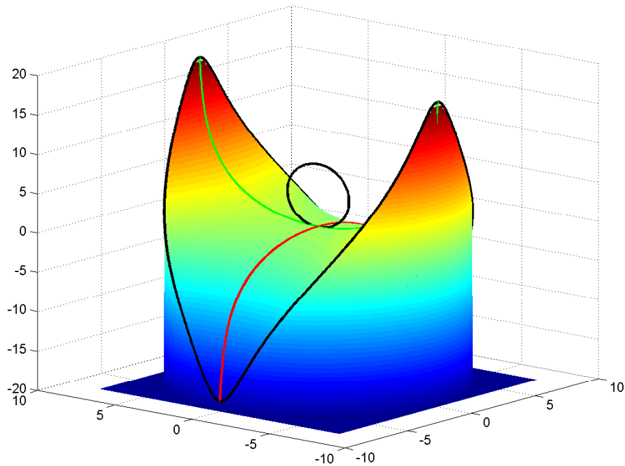
Abbildung 3: Minimalfläche über dem Kreis, mit stark verbogener Randkurve, zur Erzielung einer möglichst großen Krümmung oder eines möglichst kleinen Krümmungskreises über dem Nullpunkt
